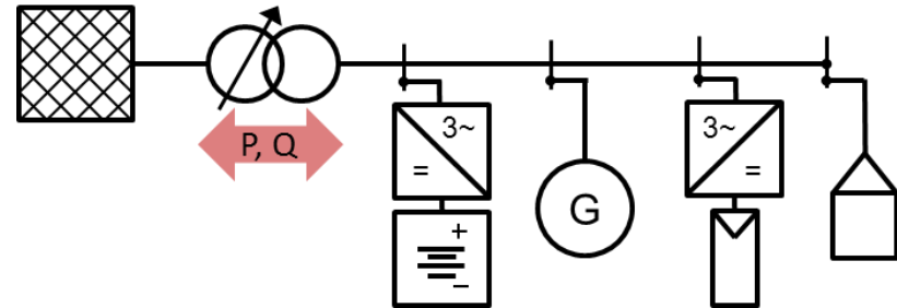
Mittelspannungsschaltanlage
